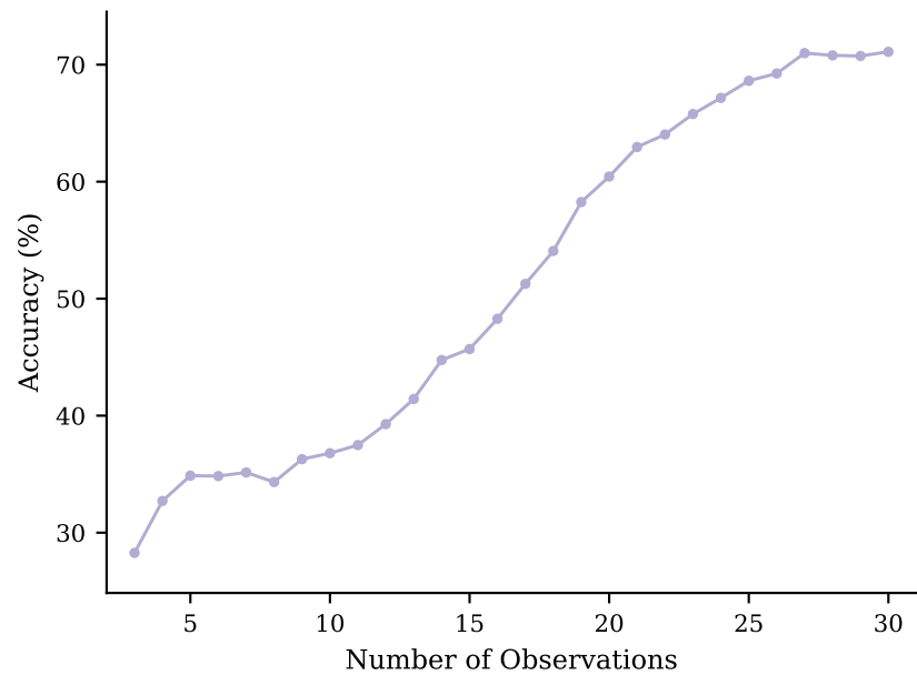
(d) E2E Transformer (no pre-training)
